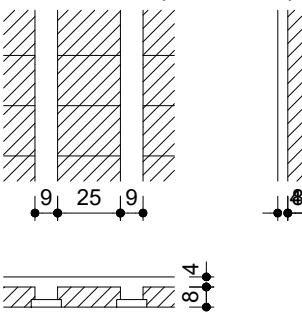
Detalhe 1 (esc. 1:30)
